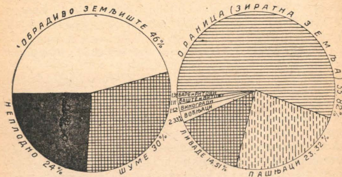
Сл. 23. — Величина разних врста земљишта.
